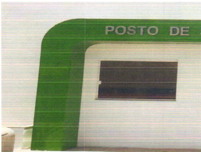
FOTO 03 - Revestimento metálico em alumínio composto (Alucobond), e=0,3mm, pintura Kaynar 500 composta por seis camadas, inclusive estrutura metálica auxiliar em perfil de viga "U" de 2" - fornecimento e montagem
